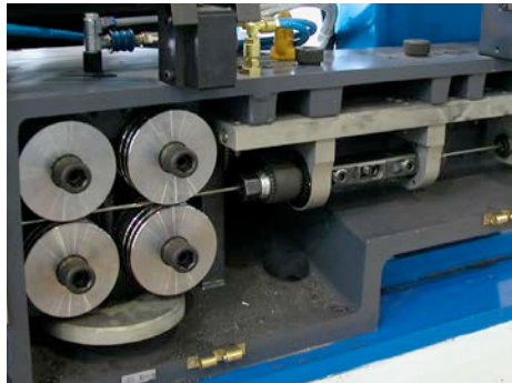
Unidad de enderezado Syrocut
